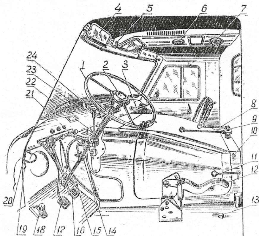
Кабина УАЗ-450.
